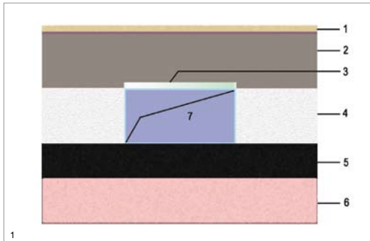
Abb. 1 Fußbodenaufbau für die Verlegung einer MINI-Luftleitung.
